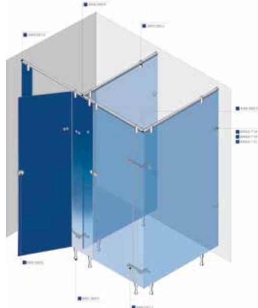
Diagrama herrajes para baño redondo
