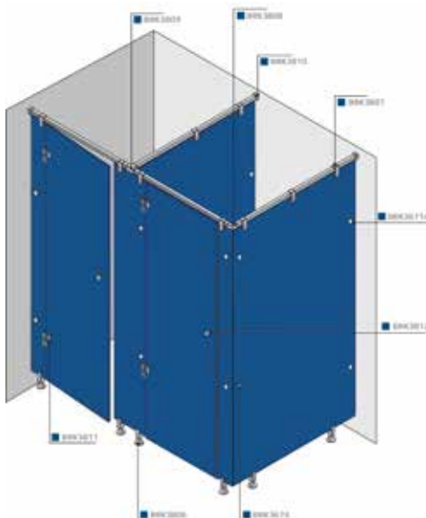
Diagrama herrajes para baño cuadrado
