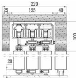
Vista transversal de la instalación general.
